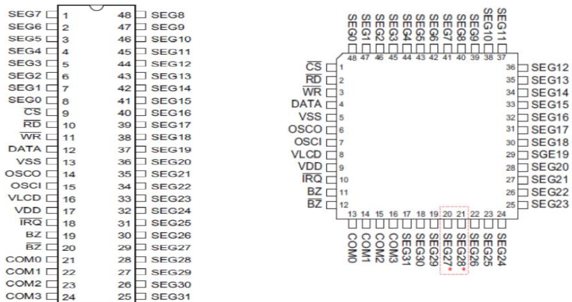
HT1621B SSOP 48
